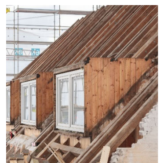
Gavl mod Vest
